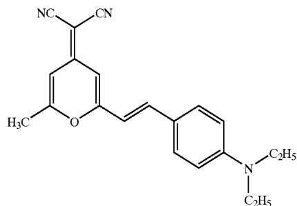
DCM-1
