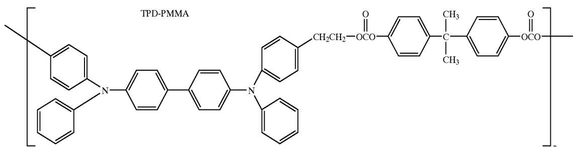
TPD-PCA
