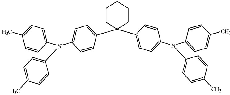
TPAC
